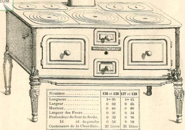
CUISINIÈRES N OS 138 et 139
